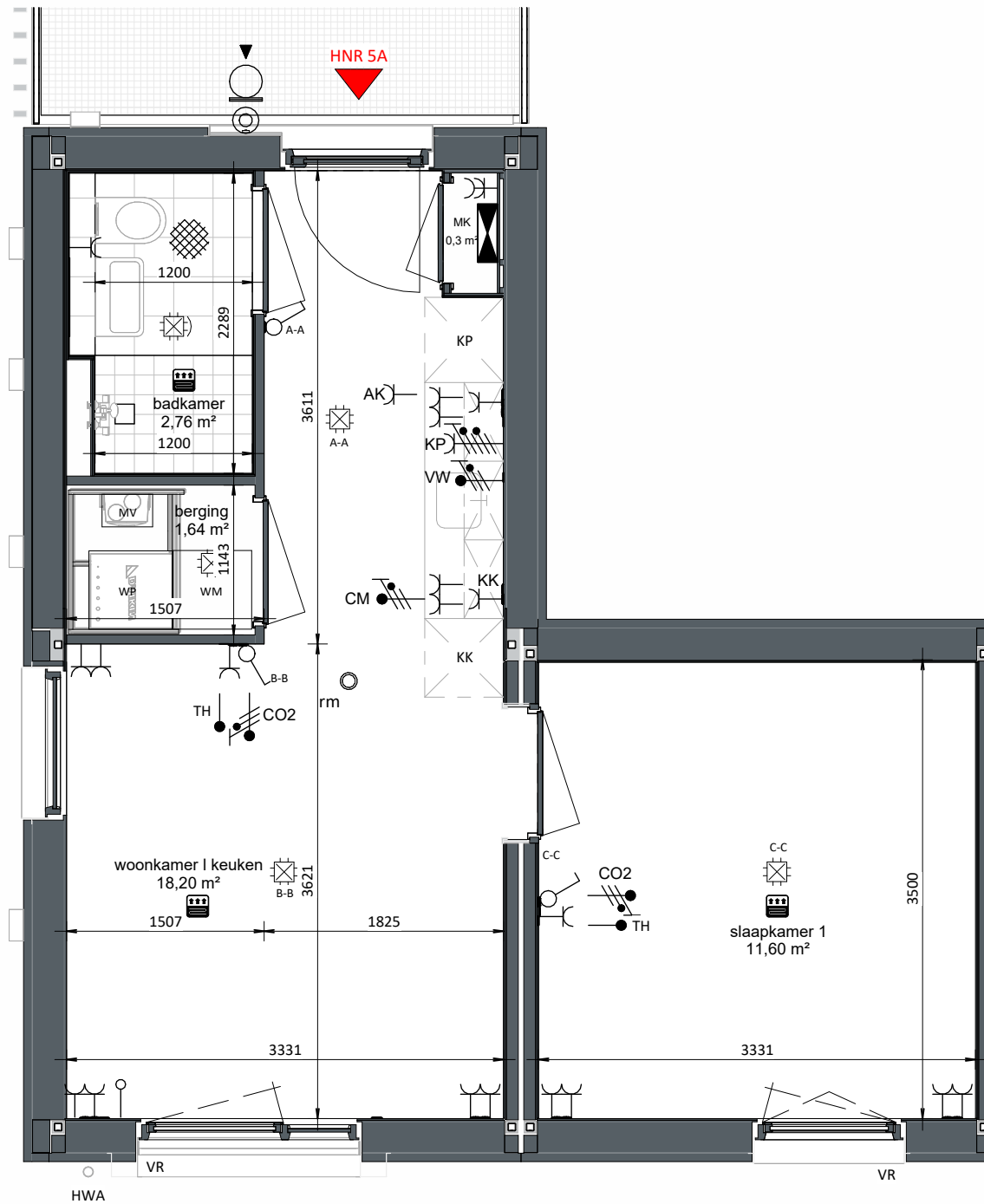
Plattegrond
