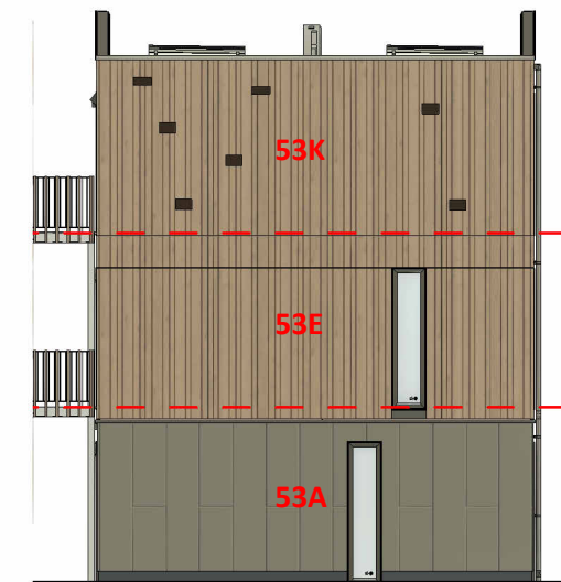
Rechterzijgevel
