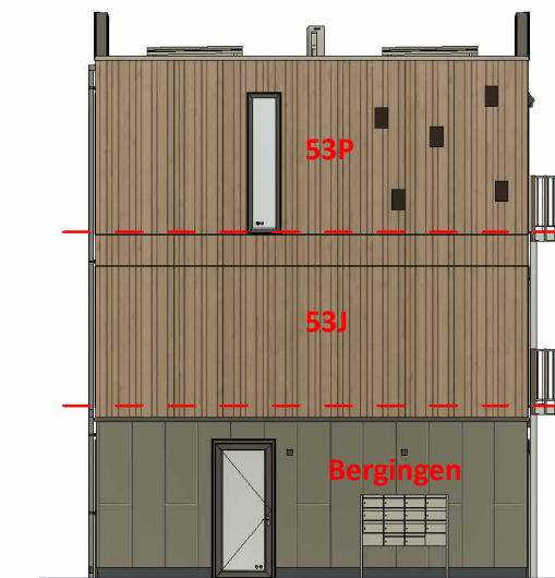
Linkerzijgevel
